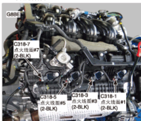
245. 发动机右侧
