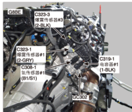
243. 发动机后部
