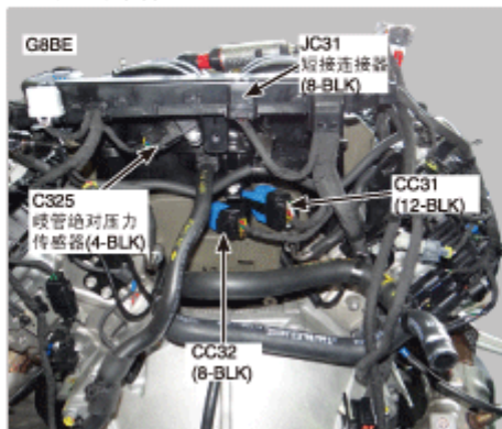
242. 发动机后部
