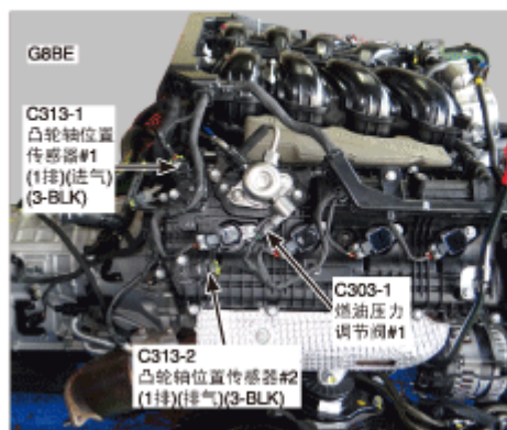
244. 发动机右侧
