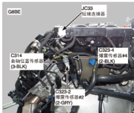
241. 发动机后部
